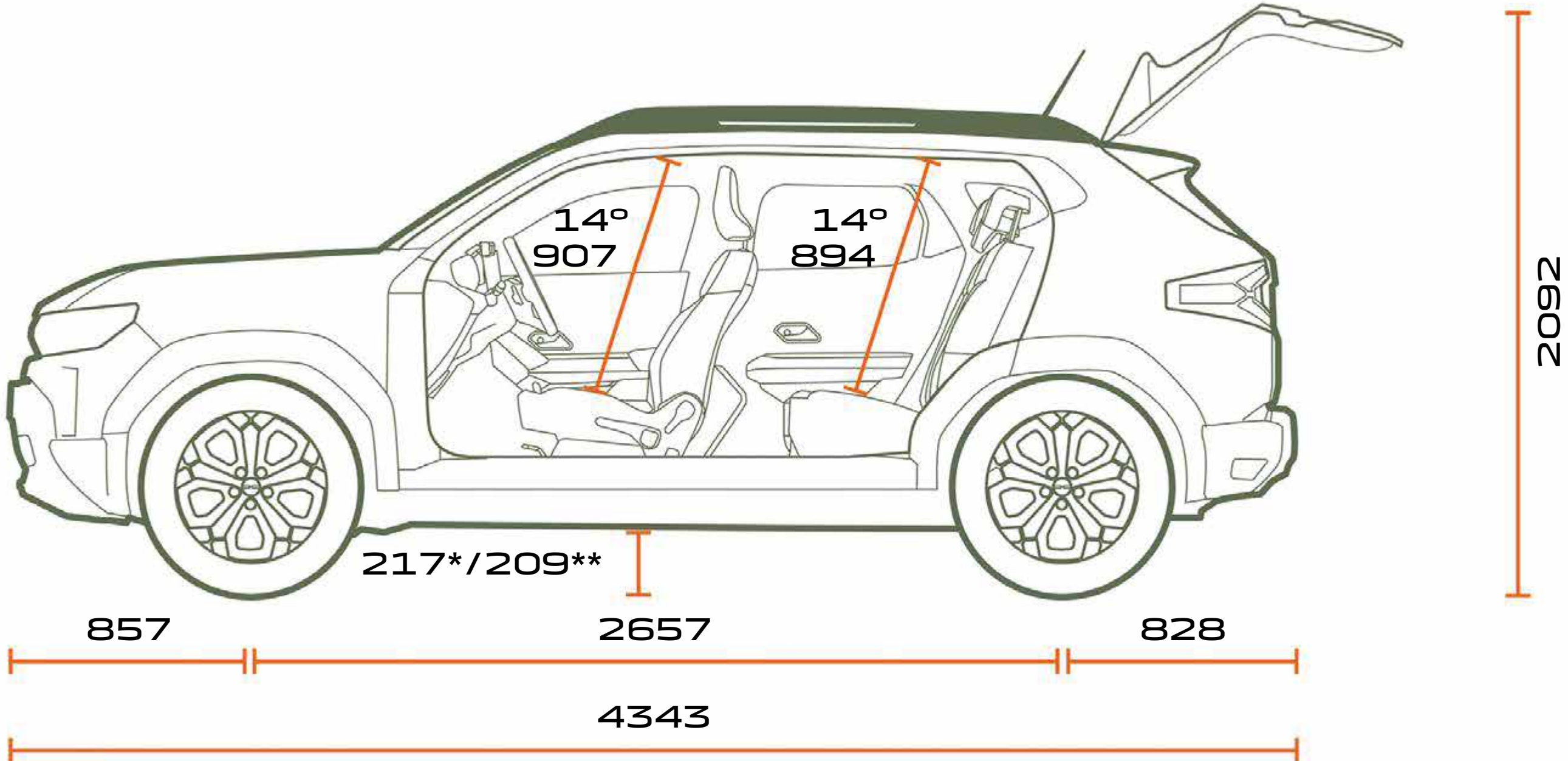
POGLED IZ PROFILA
