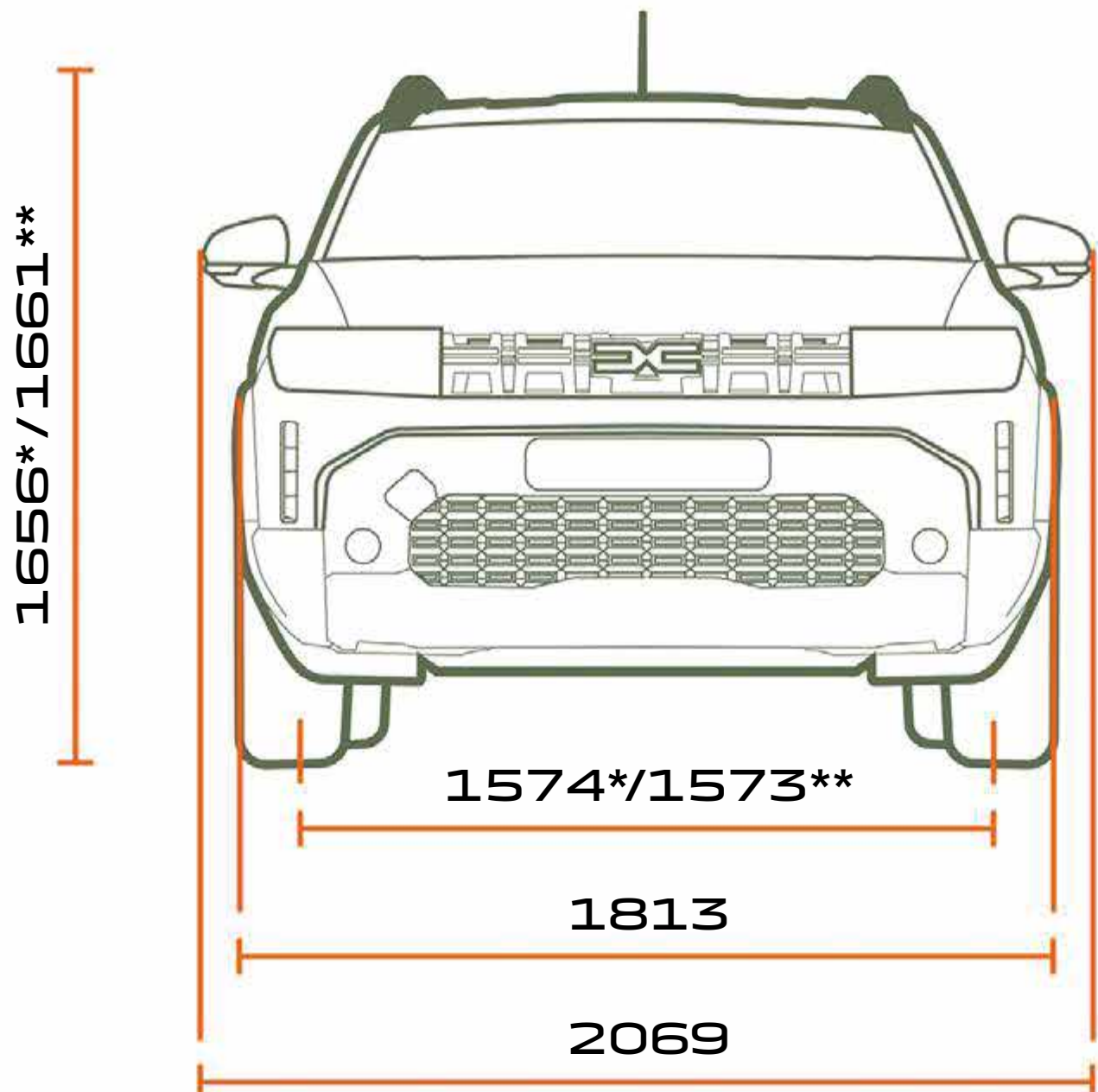
POGLED SPRIJEDA
